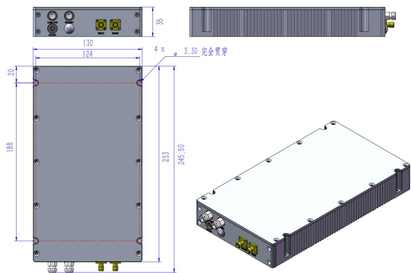
机箱尺寸图
